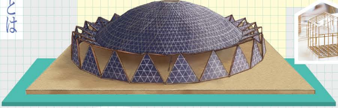
パンタドーム構法模型 / 川口衛
